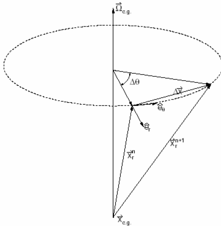
Figura 32 – Sistema de coordenadas para corpo rígido (Extraído de Fluent 6.1 User's Guide, 2003)
