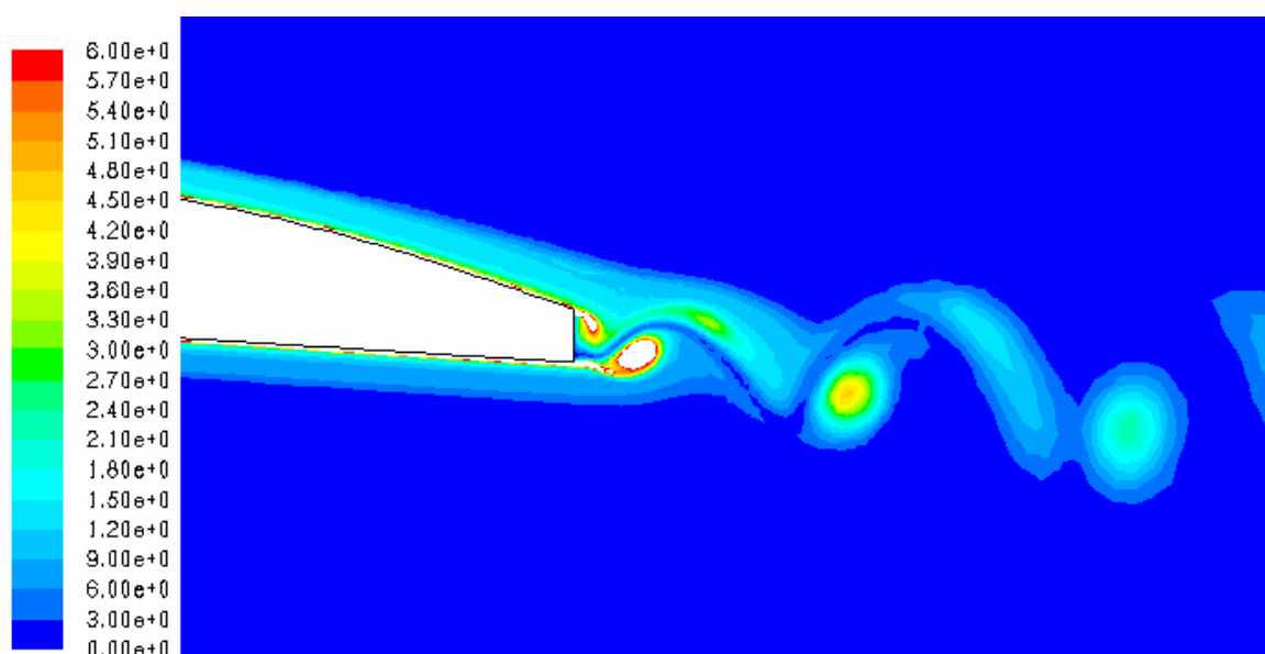
Figura 57 – Perfil 7 – Campo de Vorticidade [1/s]
