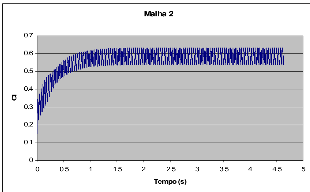
Figura 39 - Variação de CI com o tempo de simulação
