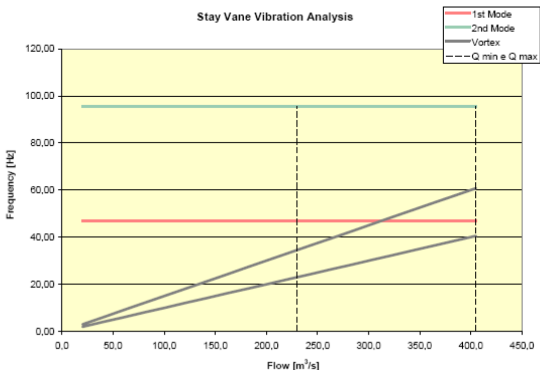
Figura 45 – Estimativa de frequência de emissão de vórtices (Extraído de [13])
