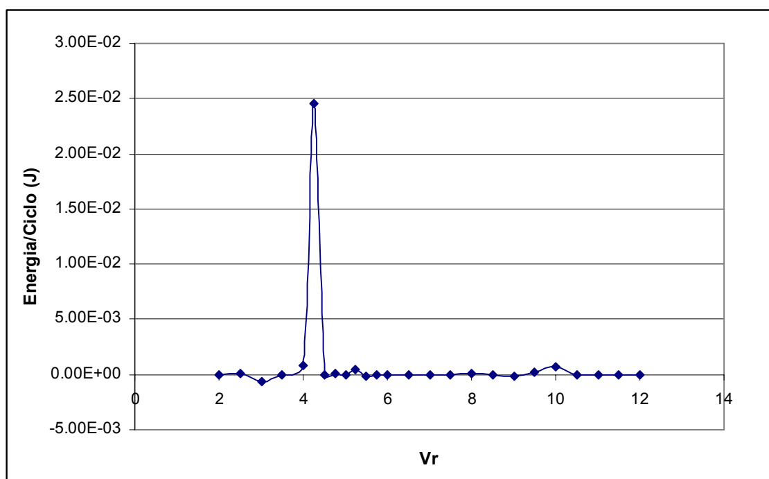
Figura 64 – Energia transferida do escoamento para a estrutura em função da Velocidade Reduzida
