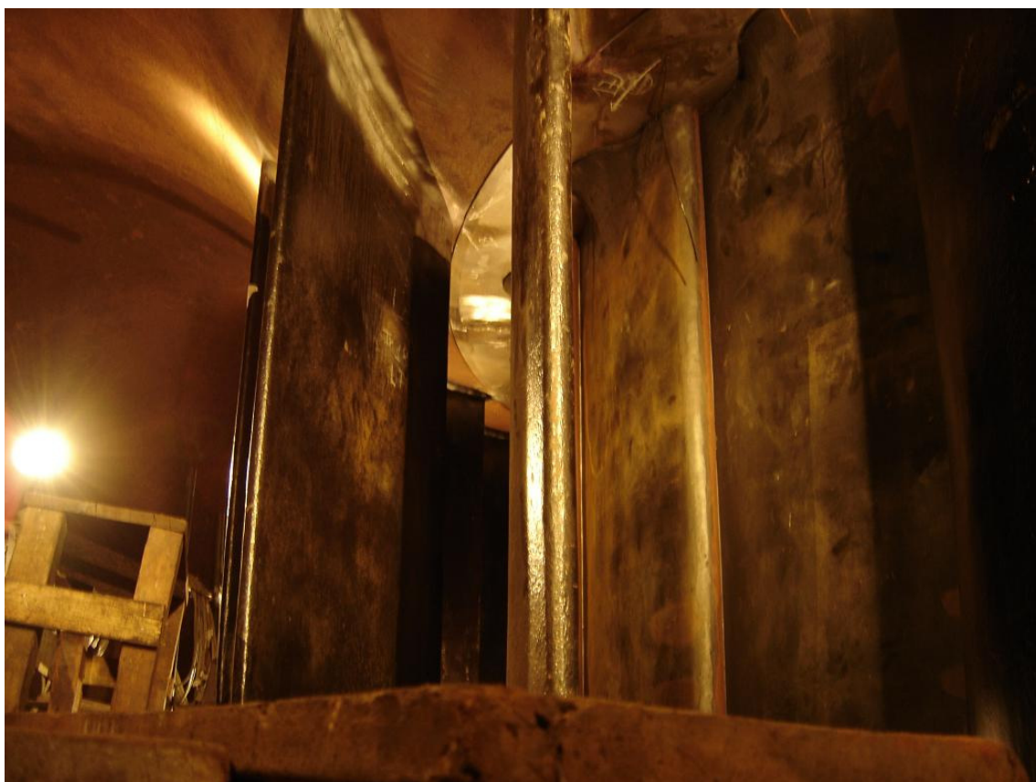
Figura 19 – Travessas da Unidade 03 de UHE Capivara com palhetas distribuidor fechadas ao fundo
