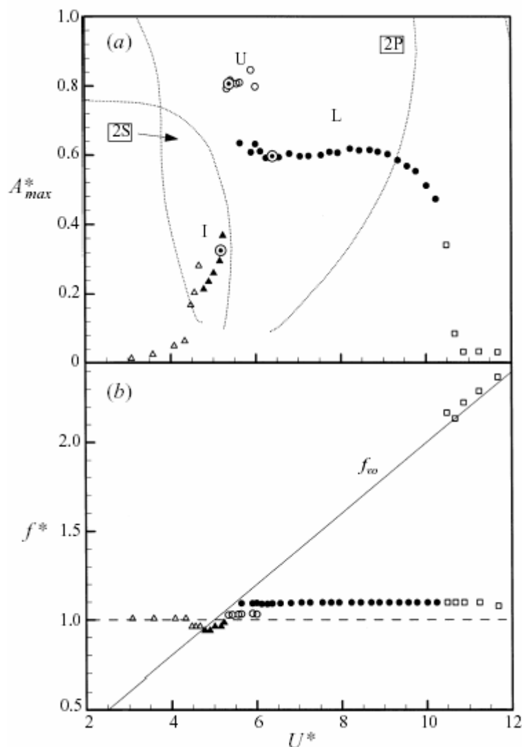
Figura 29 – Respostas de Amplitude ( A^* ) e Frequência( f^* ) em função da Velocidade Reduzida ( U^* ). Neste caso, com baixo parâmetro massa-amortecimento ( m^*\xi ), os três ramos de resposta podem ser visualizados. (Extraída de Govardhan (2000))
